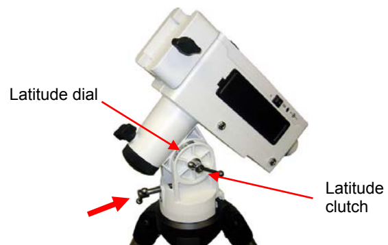
Figure 6. Adjust mount latitude
